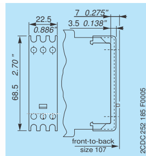
COV.01 – Plombovatelný průsvitný kryt
