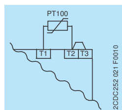
Zapojení 2-vodičového senzoru
