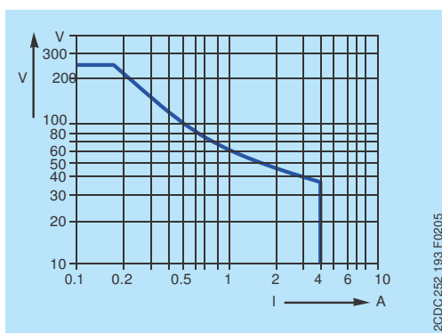
Stejnosměrná (DC) zátěž odporová
