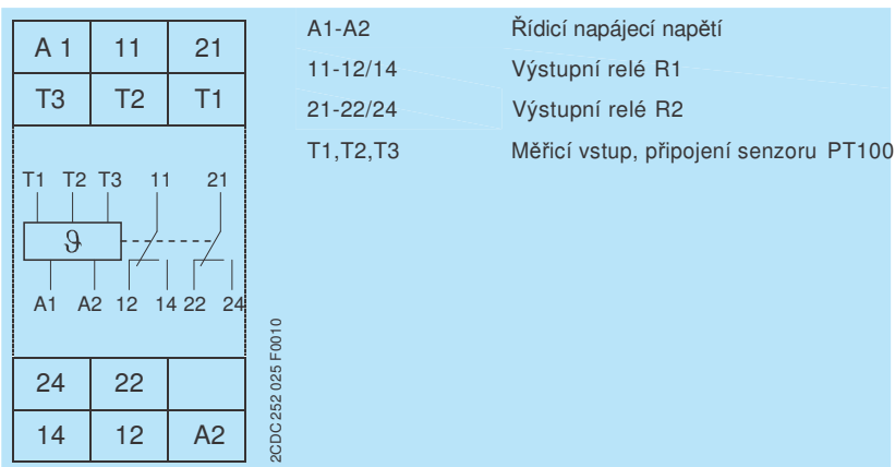
Schéma zapojení
