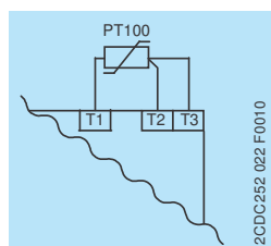
Zapojení 3-vodičového senzoru
