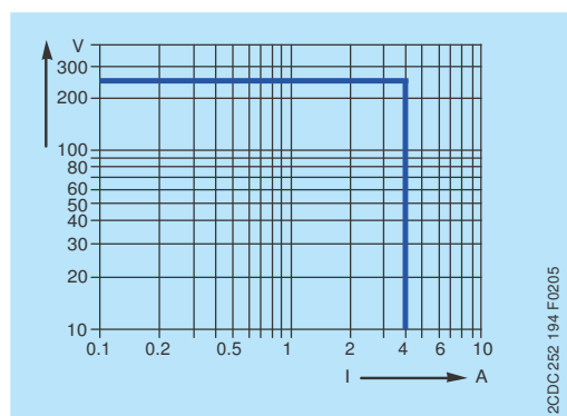
Střídavá (AC) zátěž odporová
