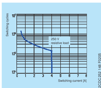
Životnost kontaktů
