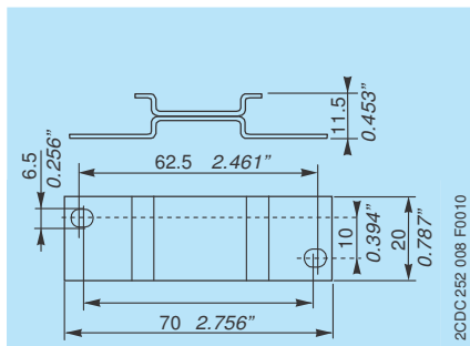
ADP.01 – Adaptér pro šroubové uchycení
