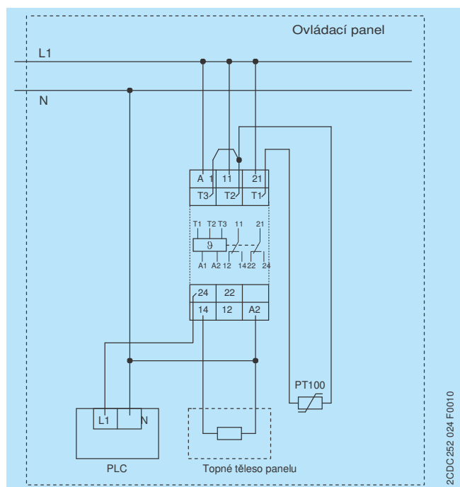
Ovládací panel, monitorování teploty
